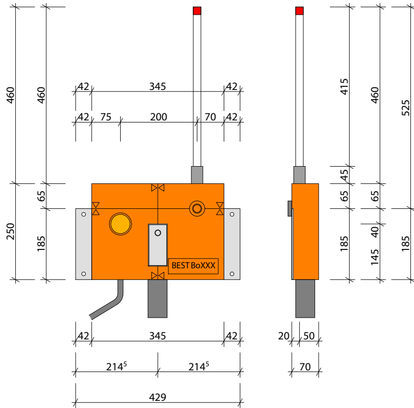
Waschmaschinen-Anschluß Trockenbau, oben
