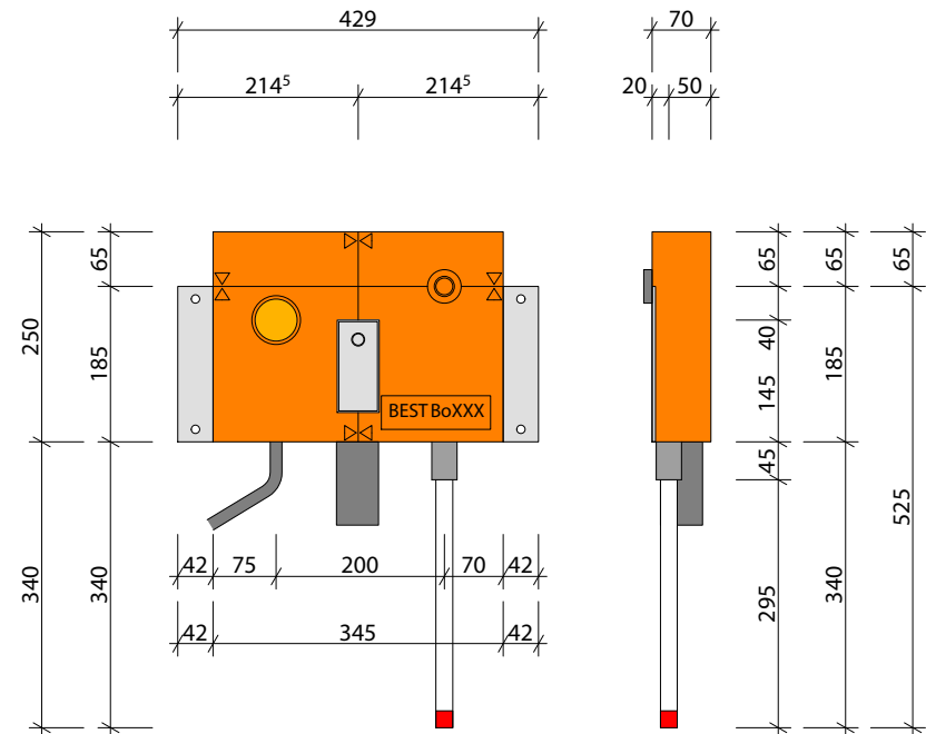
Waschmaschinen-Anschluß Trockenbau, unten
